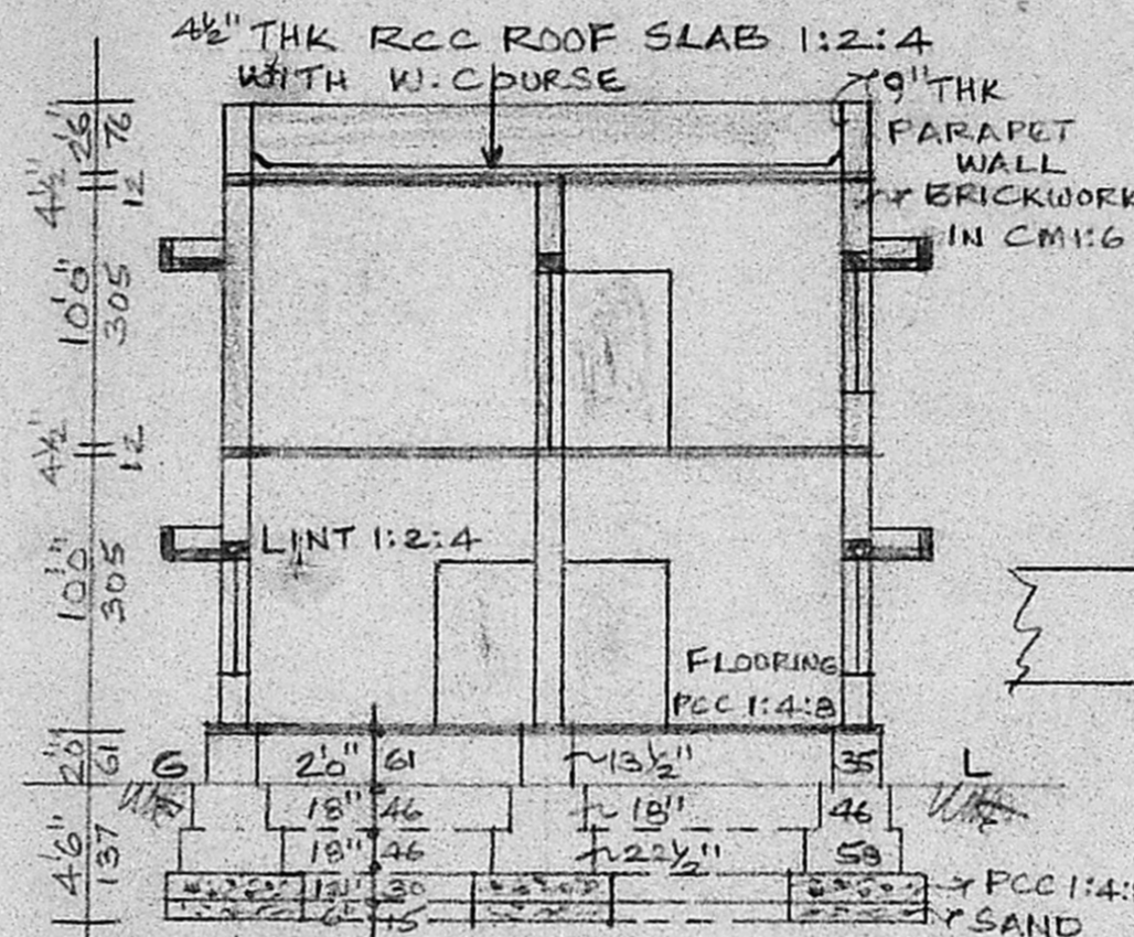
SECTION 'AB'
